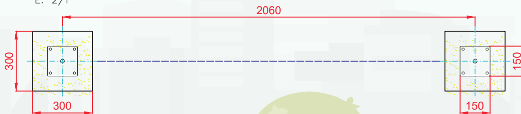
PLANTA CIMENTACIÓN E: 2/1
