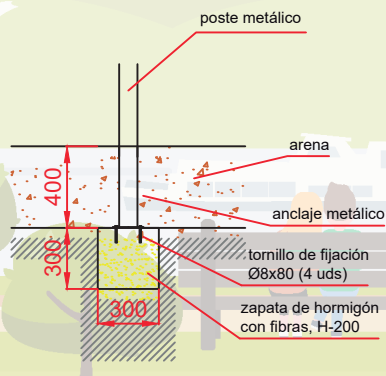
DETALLES CIMENTACIÓN ESQUEMA DE CIMENTACIÓN EN ARENA
