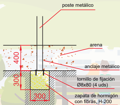
DETALLES CIMENTACIÓN ESQUEMA DE CIMENTACIÓN EN ARENA
