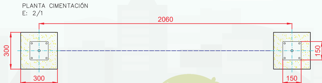
DETALLES CIMENTACIÓN ESQUEMA DE CIMENTACIÓN EN ARENA
