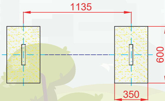
PLANTA CIMENTACIÓN
