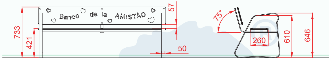
PERFIL IZQUIERDO
