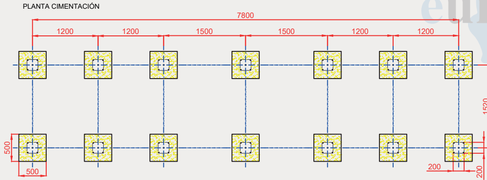
DETALLES CIMENTACIÓN ESQUEMA DE CIMENTACIÓN EN HORMIGÓN E: 2/1
