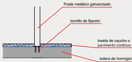
DETALLES CIMENTACIÓN ESQUEMA DE CIMENTACIÓN EN HORMIGÓN E: 2/1
