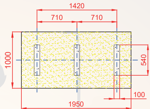
PLANTA CIMENTACIÓN
