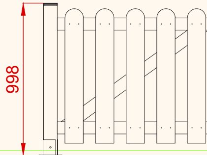
ALZADO
