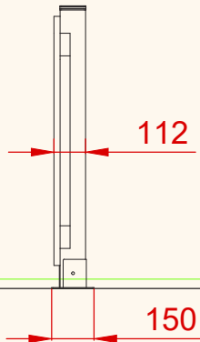
PERFIL DERECHO
