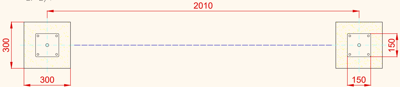
PLANTA CIMENTACIÓN E: 2/1
