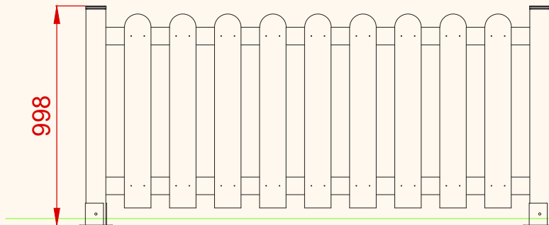
ALZADO
