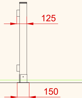
PERFIL IZQUIERDO
