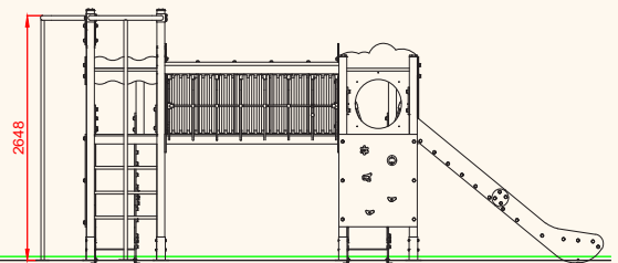
PERFIL IZQUIERDO
