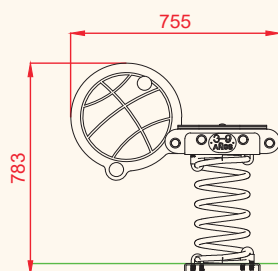
ALZADO
