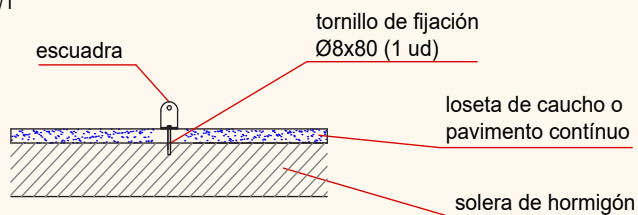
ESQUEMA DE CIMENTACIÓN EN HORMIGÓN E: 2/1
