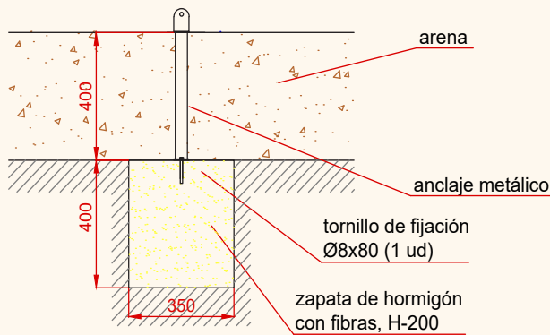
ESQUEMA DE CIMENTACIÓN EN ARENA E: 2/1
