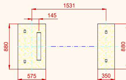
PLANTA CIMENTACIÓN
