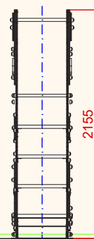
PERFIL IZQUIERDO
