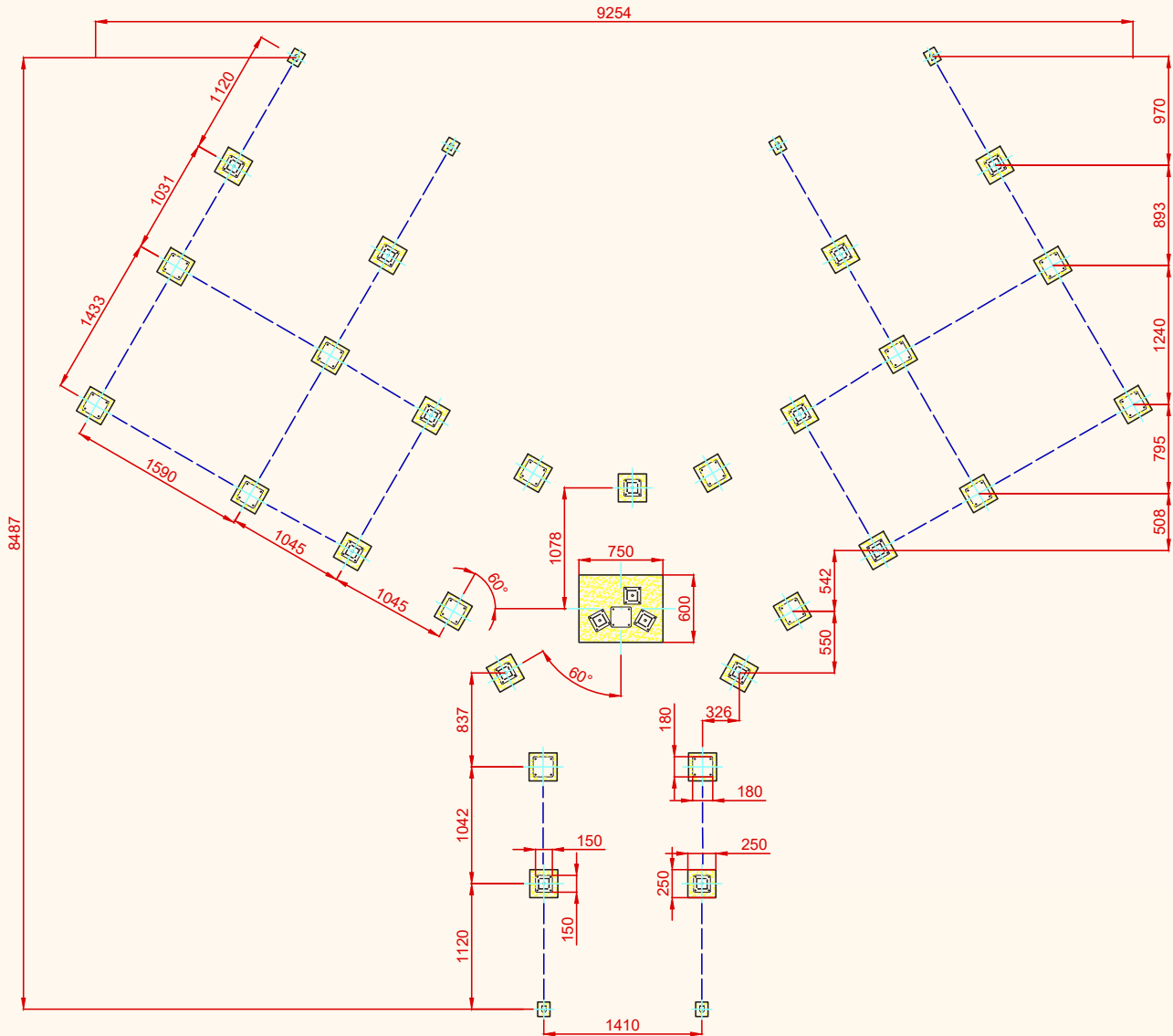
PLANTA CIMENTACIÓN
