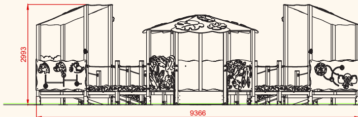
ALZADO
