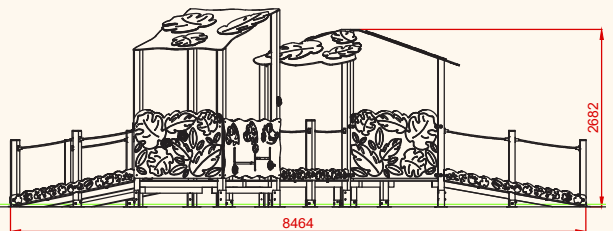
PERFIL IZQUIERDO
