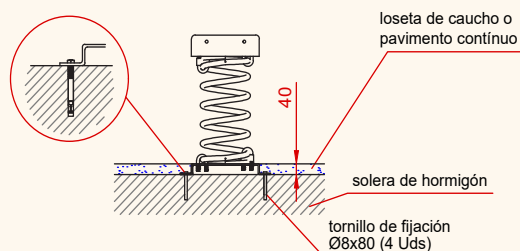
Detalle de sujeción de espirro metálico
