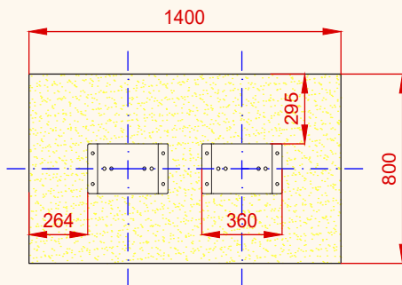
PLANTA CIMENTACIÓN
