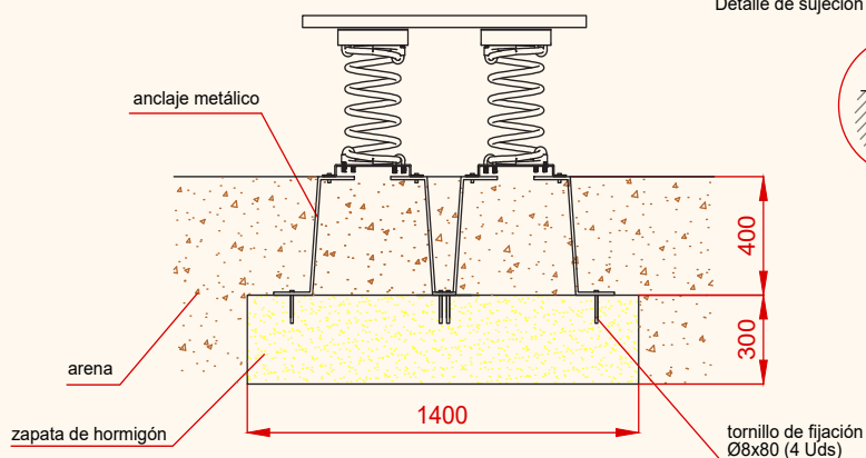
Detalle de sujeción de espirro metálico
