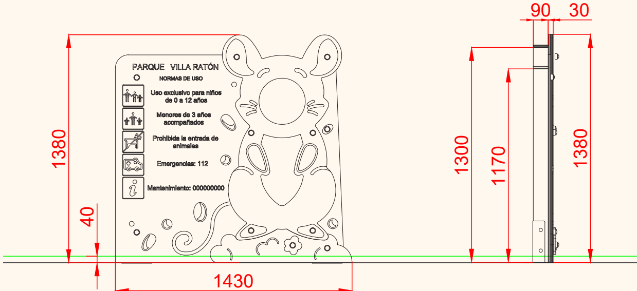
ALZADO
