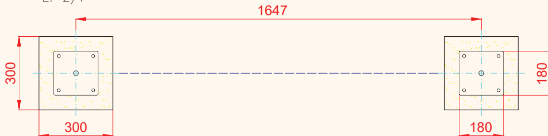
PLANTA CIMENTACIÓN E: 2/1
