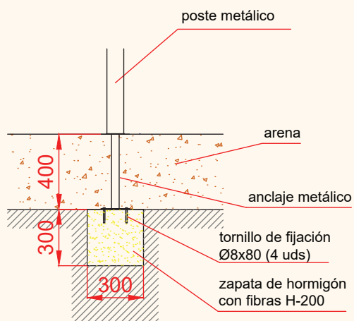
DETALLES CIMENTACIÓN ESQUEMA DE CIMENTACIÓN EN ARENA
