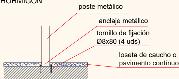
ESQUEMA DE CIMENTACIÓN EN HORMIGÓN
