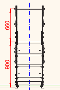
PERFIL
