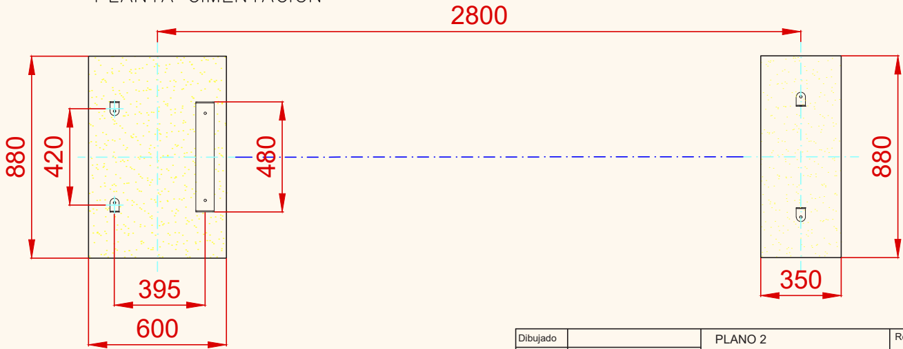
PLANTA CIMENTACIÓN
