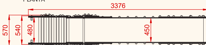
PLANTA
