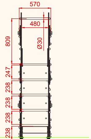
PERFIL
