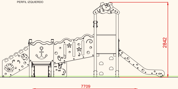
PERFIL IZQUIERDO
