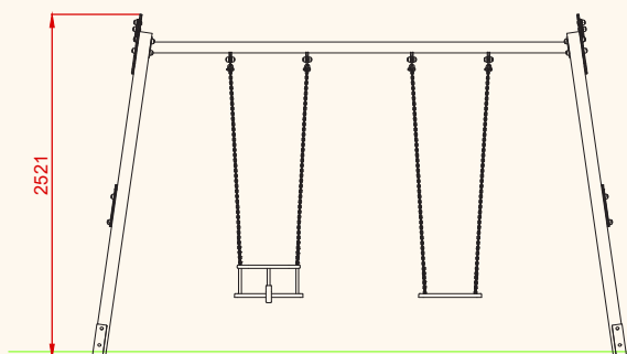
ALZADO
