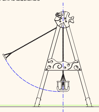
PERFIL IZQUIERDO
