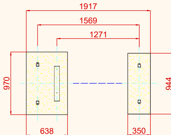
PLANTA CIMENTACIÓN
