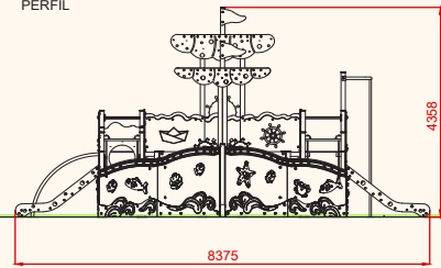
PERFIL
