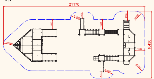
ÁREA DE SEGURIDAD Superficie= 170,27 m 2 E1/2
