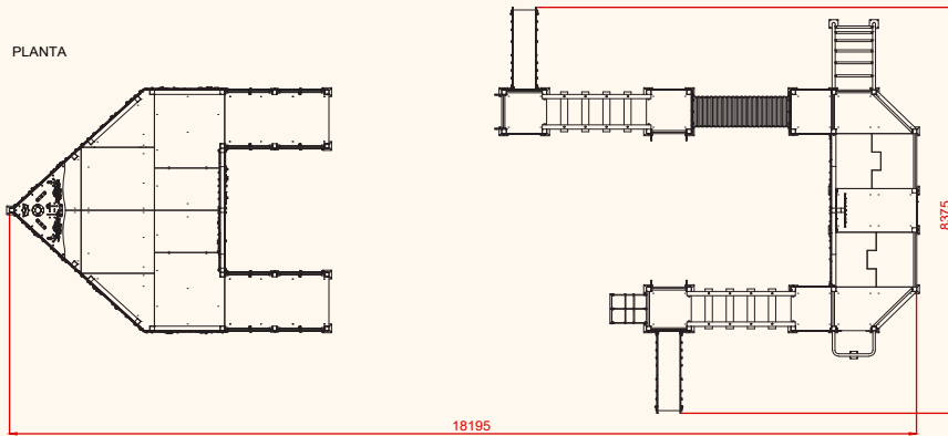
ÁREA DE SEGURIDAD Superficie= 170,27 m 2 E1/2
