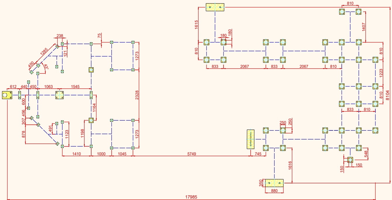
PLANTA CIMENTACIÓN
