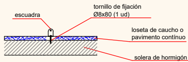
ESQUEMA DE CIMENTACIÓN EN HORMIGÓN
