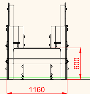
PERFIL IZQUIERDO
