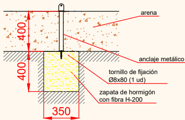
ESQUEMA DE CIMENTACIÓN EN ARENA
