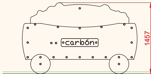
ALZADO
