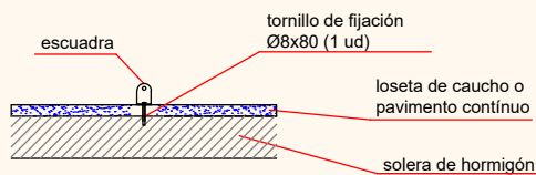
ESQUEMA DE CIMENTACIÓN EN HORMIGÓN
