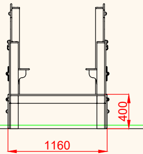
PERFIL IZQUIERDO
